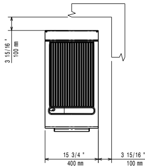
Felülnézet
