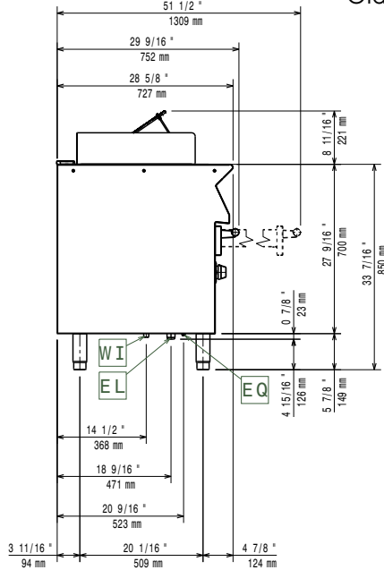
Oldalnézet
